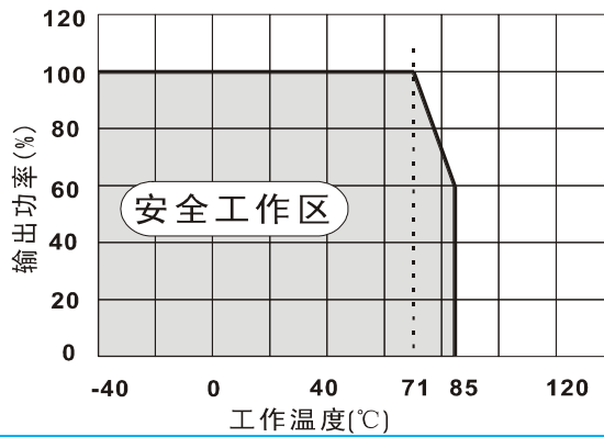
温度曲线图
