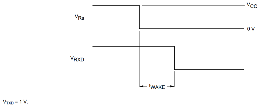
图 5 从待机状态唤醒时序图
