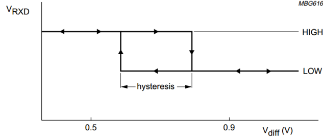
图 4 迟滞
