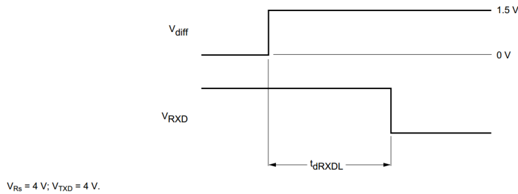
图 6 总线显性到 RXD 输出低时序图
