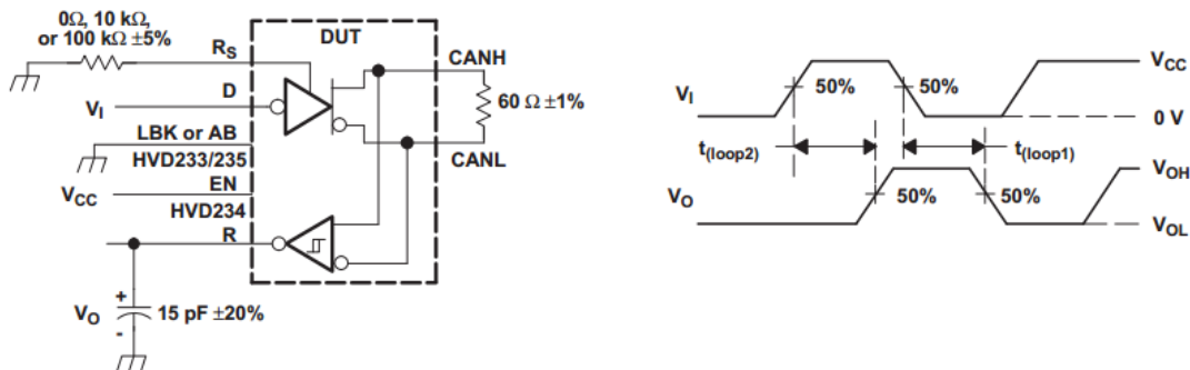
图 8 t_{\text{WAKE}} 测试电路与电压波形（休眠）
